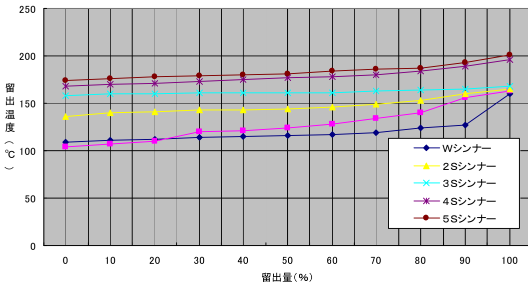
蒸留曲線
