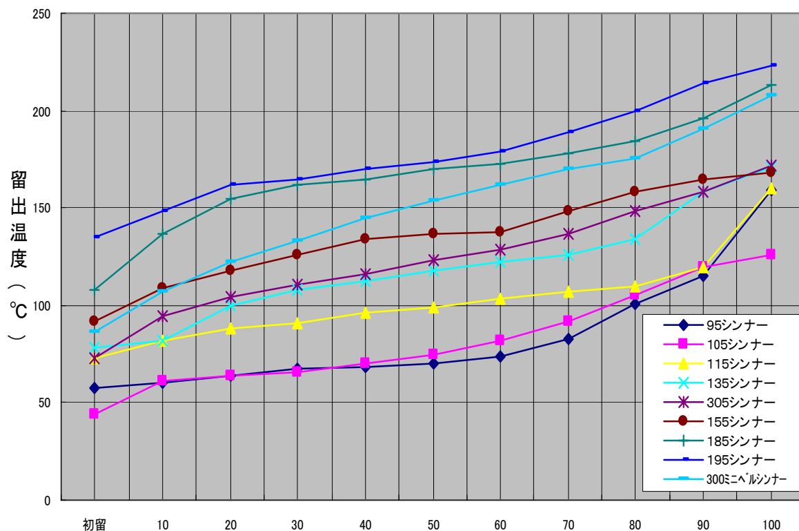
蒸留曲線
